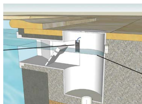
Plaatsing van de sonde in de skimmer
